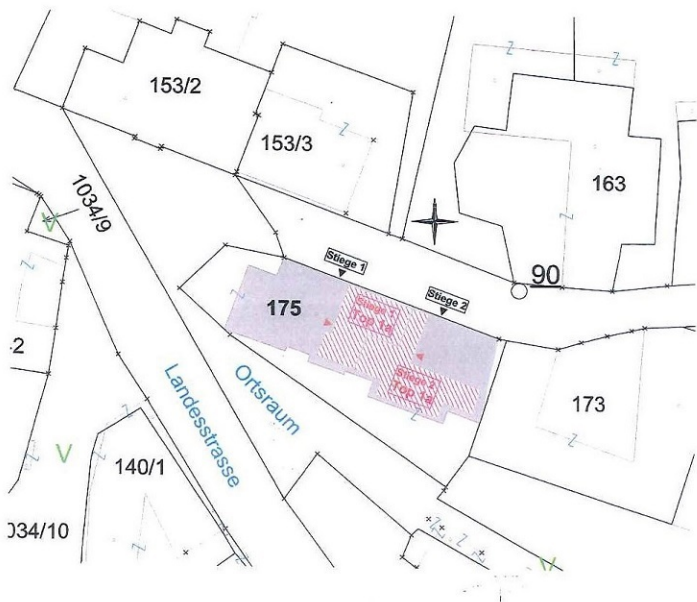
Lageplan M 1:500
