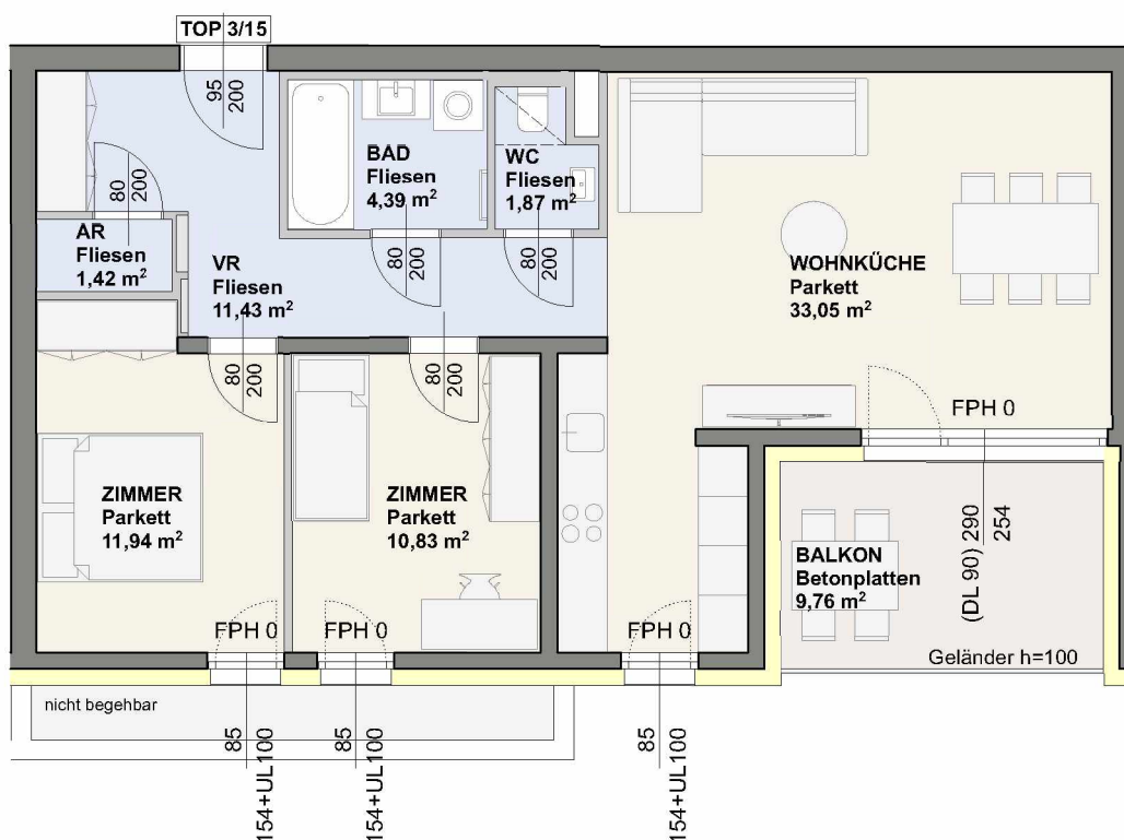
DACHGESCHOSS 1:100
