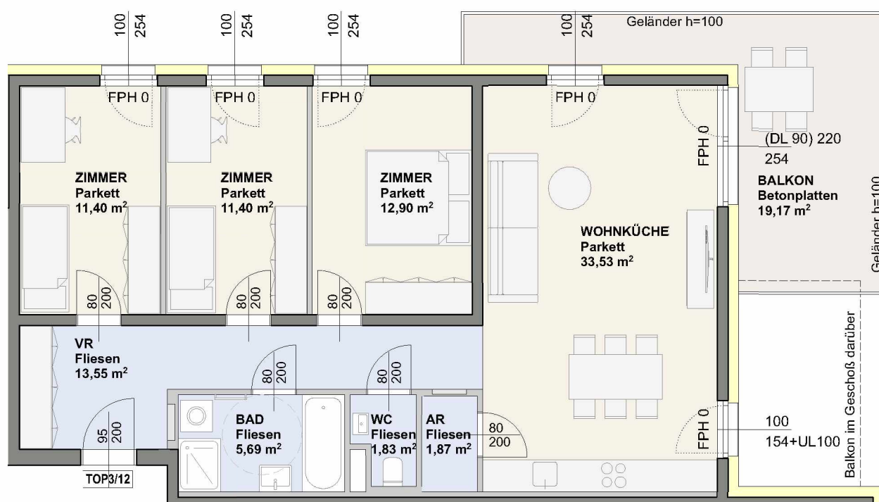
1. OBERGESCHOSS 1:100
