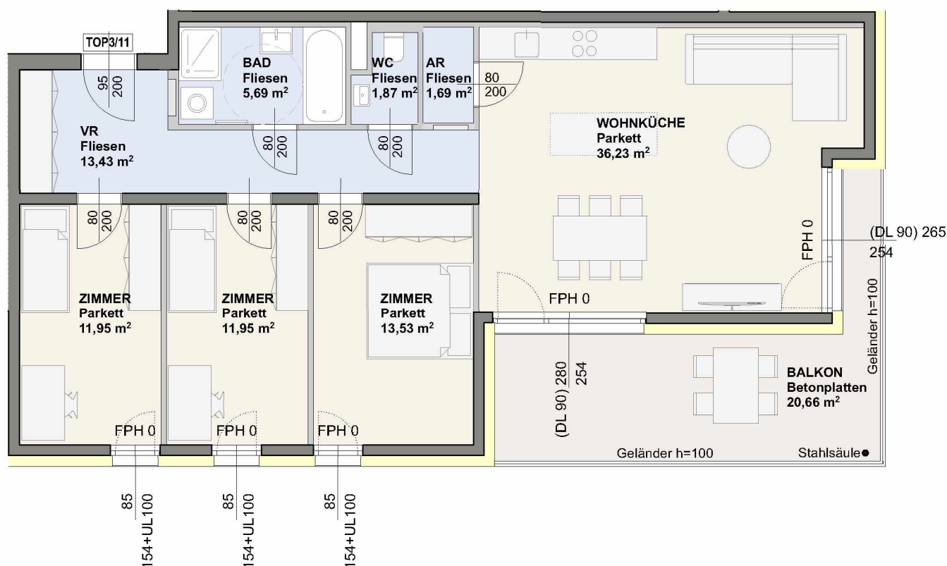
1. OBERGESCHOSS 1:100
