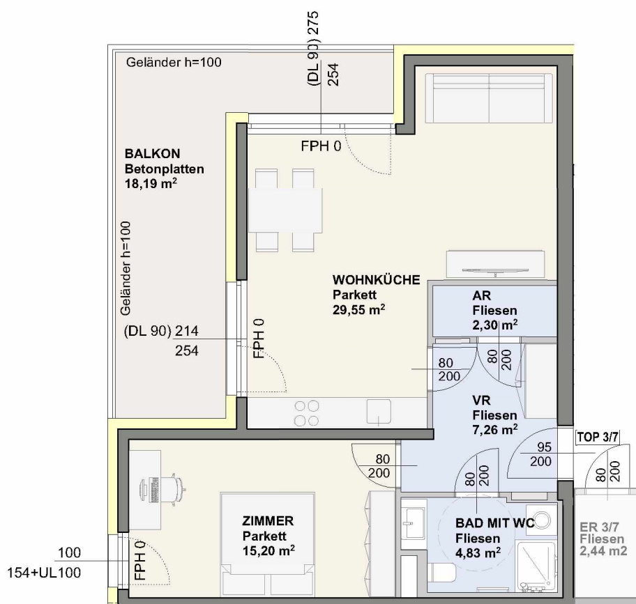
1. OBERGESCHOSS 1:100
