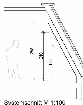
Systemschnitt M 1:100
