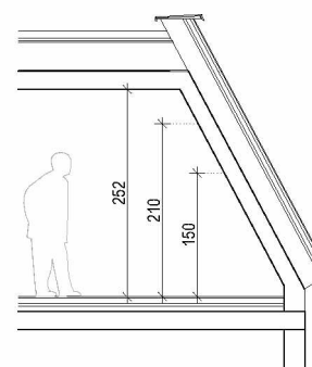
Systemschnitt M 1:100
