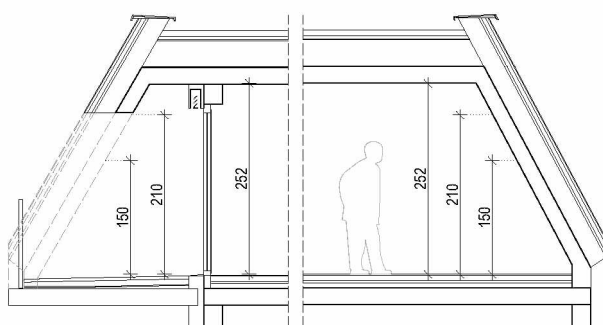
Systemschnitt M 1:100
