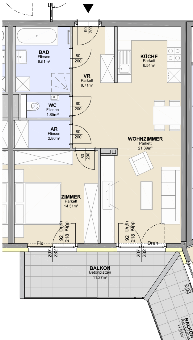
2. OBERGESCHOSS
